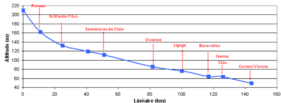
Figure 6 : Profil en long du Clain d'après SCAN 25 de l'IGN
