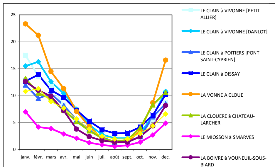
Figure 37: Débit moyen mensuel en l/s/km 2 (débit spécifique) – Banque hydro
