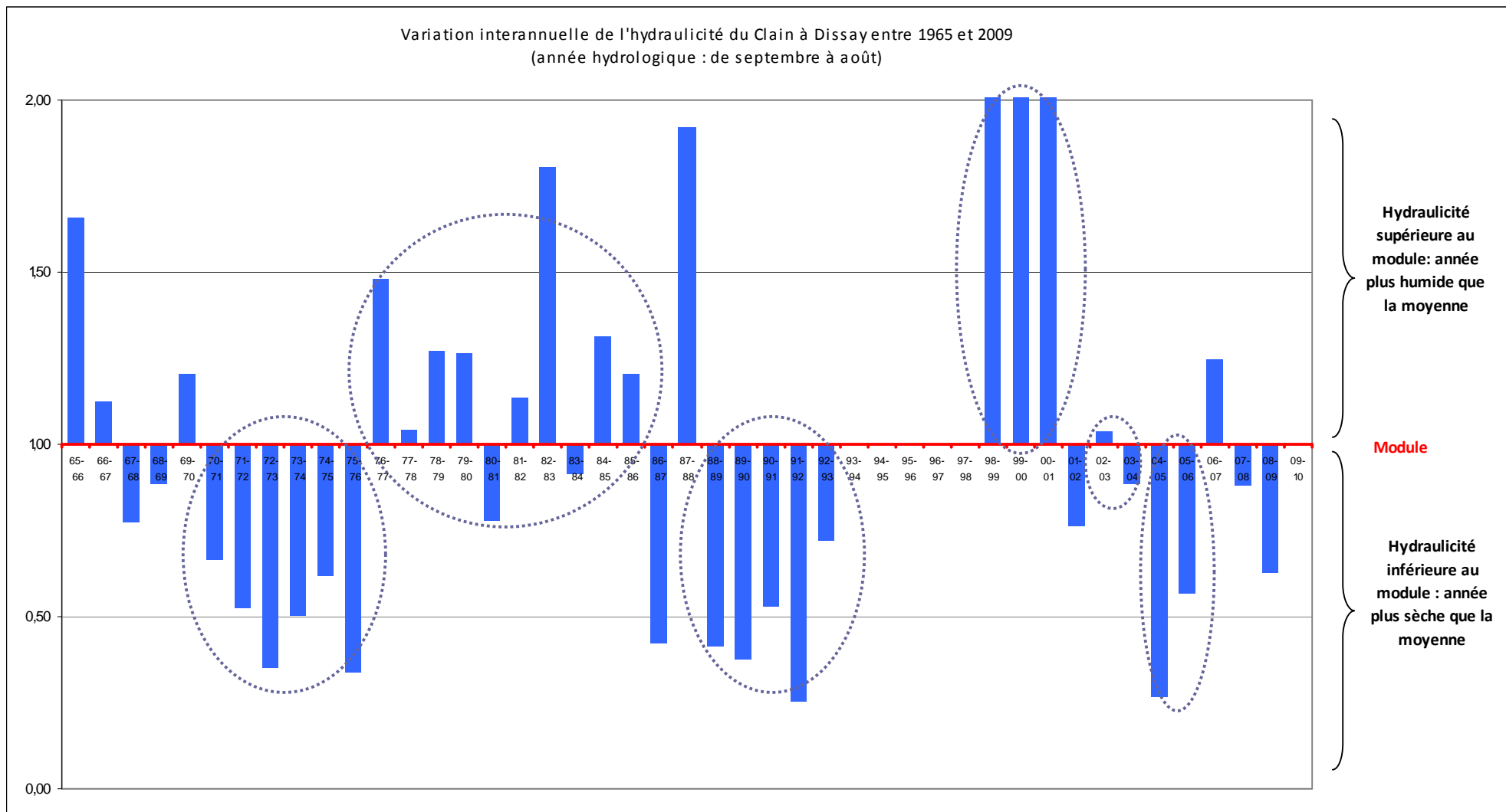
Figure 38 : Variation interannuelle de l'hydraulicité du Clain à Dissay Source: banque hydro (les données de 1993 à 1997 ne sont pas disponibles)
