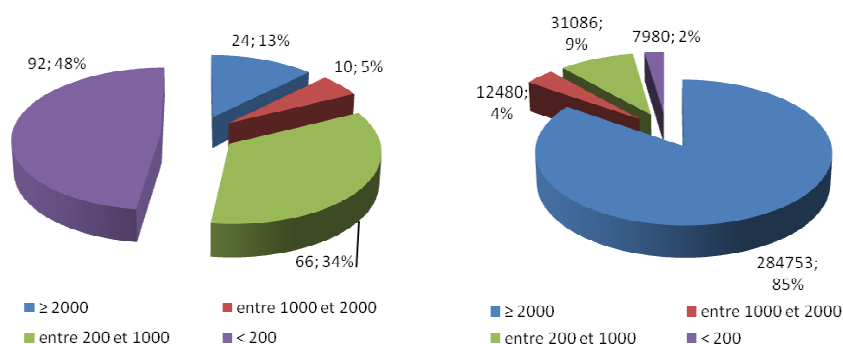
Figure 61: Nombre d'ouvrages (à gauche) et capacité épuratoire (à droite) par tranche de capacité (en Equivalent-Habitant)
