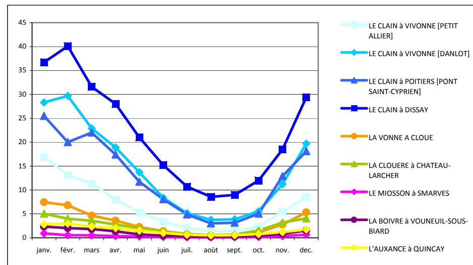
Figure 36: Débits moyens mensuels en m 3 /s – Banque hydro
