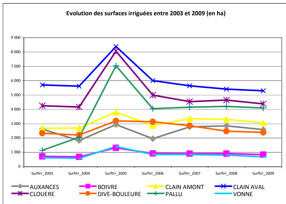
Figure 70: Evolution des surfaces irriguées entre 2003 et 2009 par sous-bassin sur la partie Vienne du bassin du Clain
