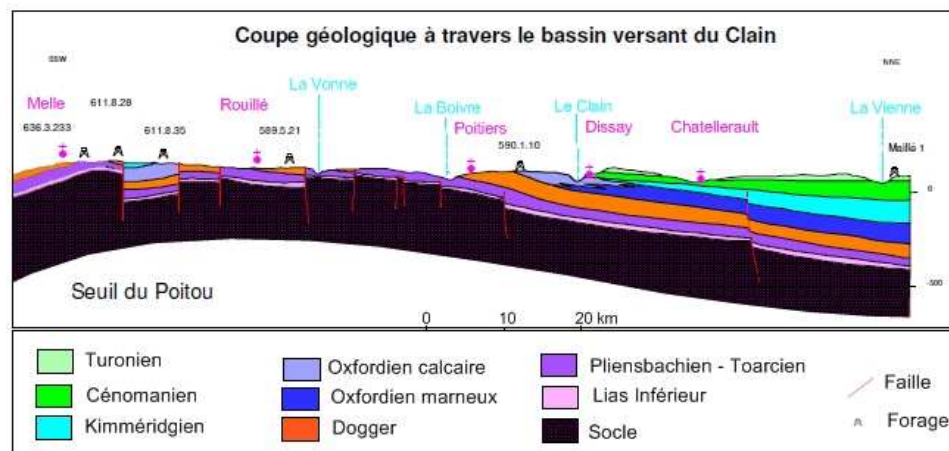
Figure 7 : Coupe géologique d'orientation SSW-NNE à travers le bassin du Clain Source : BRGM
