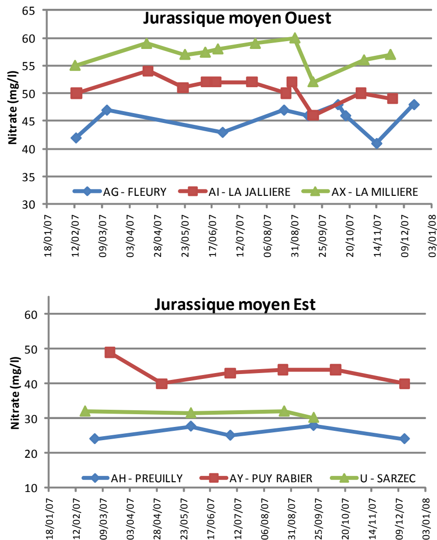
Figure 22: Exemple d'évolution saisonnière des teneurs en nitrates sur la nappe libre du Dogger en rive droite (Est) et en rive gauche (Ouest) du Clain
