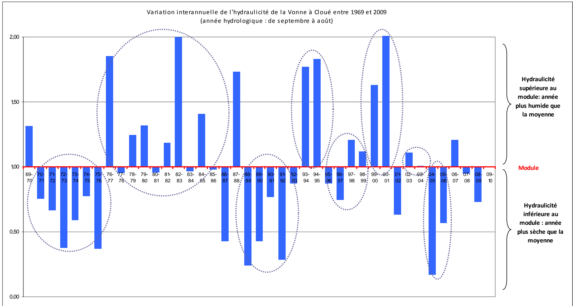
Figure 39: Variation interannuelle de l'hydraulicité de la Vonne
