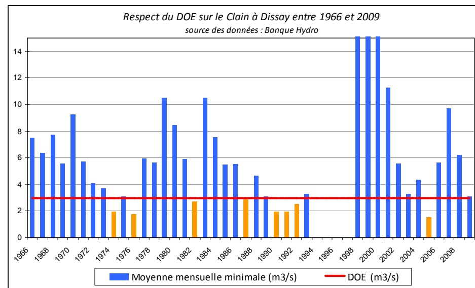
Figure 42: Respect du DOE sur le Clain à Dissay entre 1966 et 2009 Source des données : banque hydro
